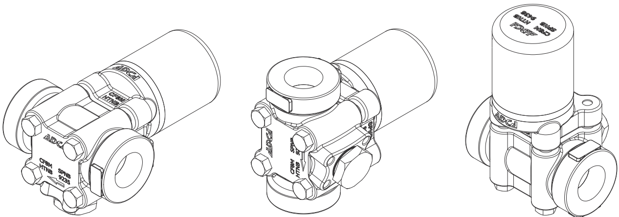
UCX90 유니버설 파이프라인 커넥터에 연결된 UBS90 스팀 트랩
