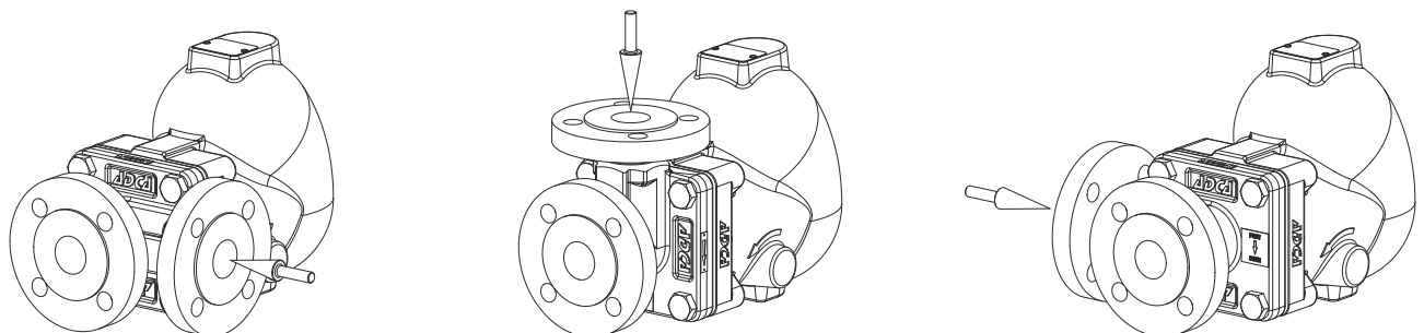
AR - 앵글 (우→전면) AL - 앵글 (좌→전면) AT - 앵글 (상→전면)
