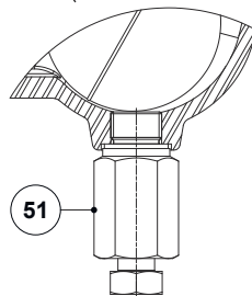
자동 선택사양 블로다운 밸브(BDV);
