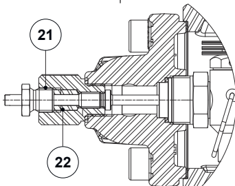
수동 선택사양 스팀 록 릴리스 (SLR)
