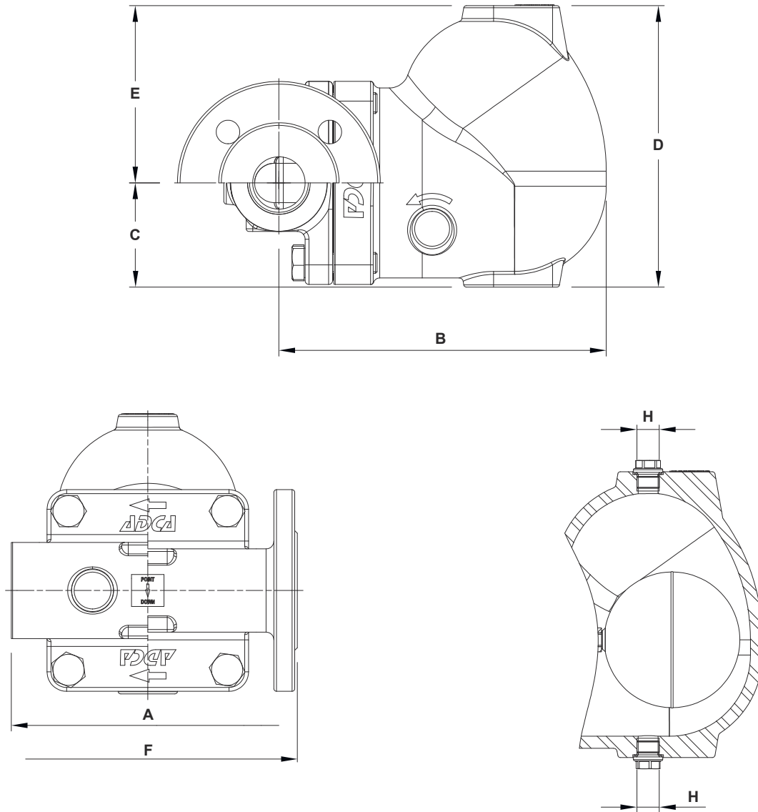
치수 (mm)
