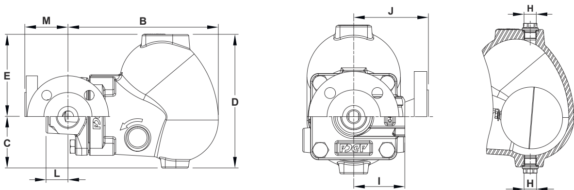
앵글형 설계
