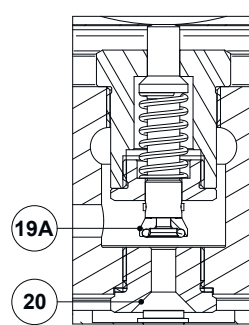
상세 A 파일럿 밸브(연질)
