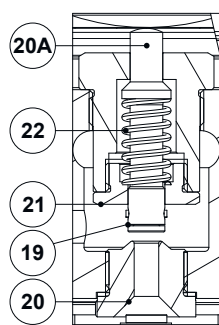
상세 A 파일럿 밸브
