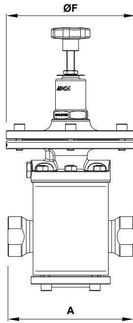
선택사양 저압 다이어프램
