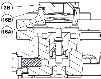
선택사양 돔 로딩
