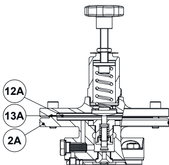
선택사양 저압 다이어프램
