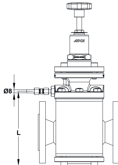
선택 외부 감지 라인 연결부
