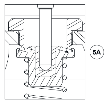
상세 B 메인 밸브(연질)
